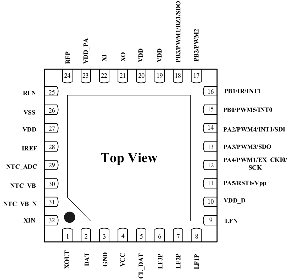
图 1-1 管脚信息图(QFN32-5x5 mm 封装)
